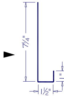
DOOR JAMB DJ-01
