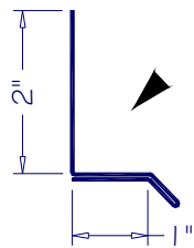
HEADER HD-01
