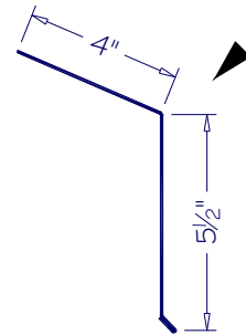
EAVE EV-04
