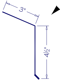
EAVE EV-03
