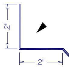
HEADER HD-02
